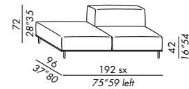
elemento penisola - peninsula unit 195
