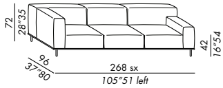
terminale angolo - corner end unit 270
