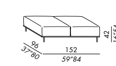
elemento isola - island unit 155
