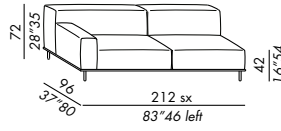
terminale - end unit 215
